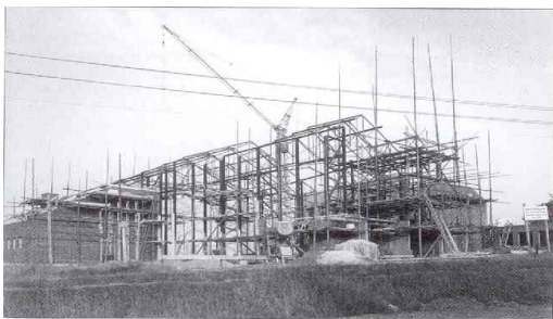
Bild des Stahlgerüsts der St. Bernward Kirche
